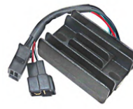
918253 Regulador Retificador SUZUKI YES 125/INTRUDER - BHD
